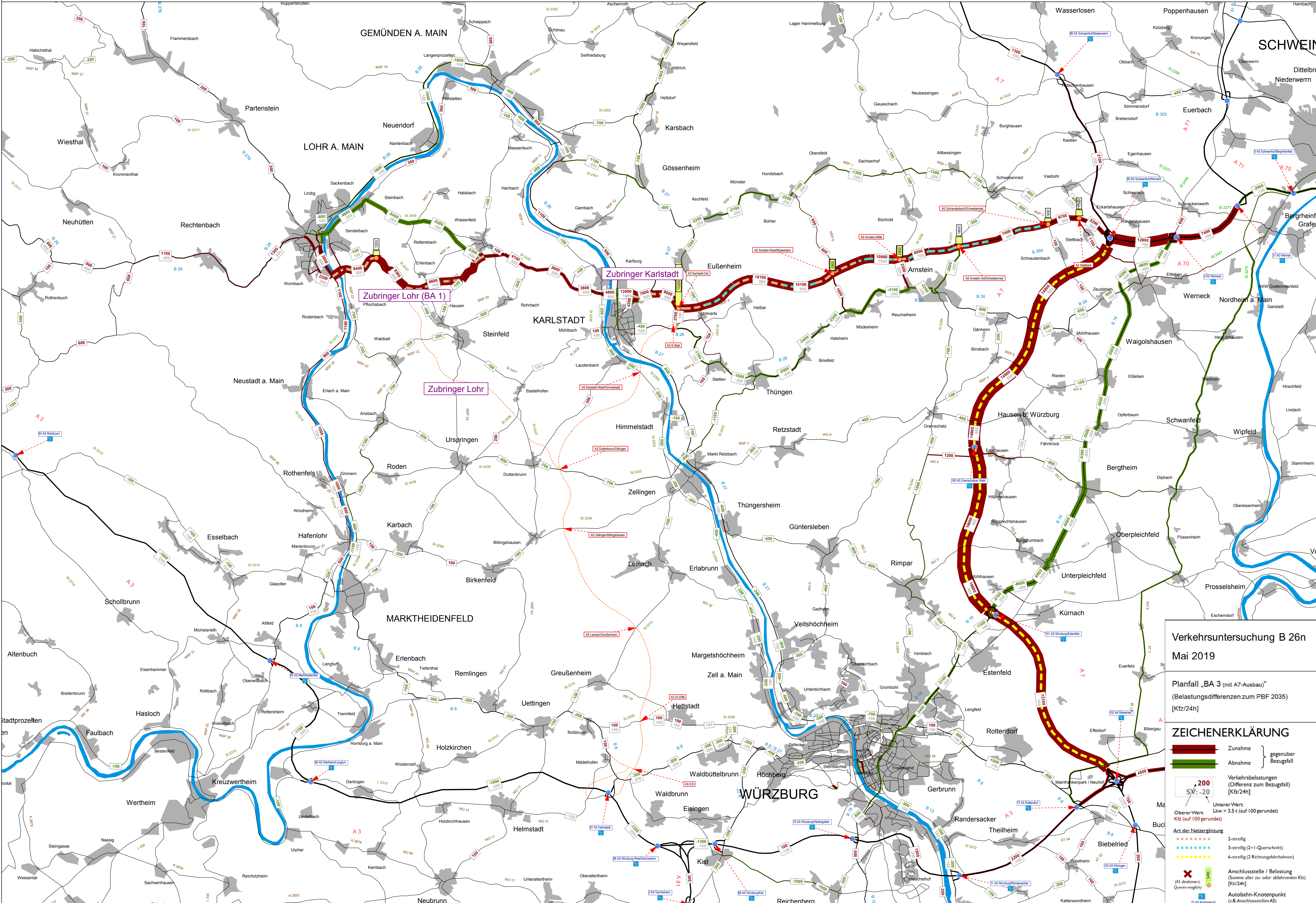
Planfall "BA 3 (mit A7-Ausbau)" (Belastungsdifferenzen zum PBF 2035) - DTV [Kfz/24h]
